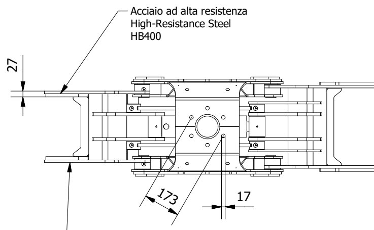
PINZA IT1500PFP 4 Punte aperte - Open tips
